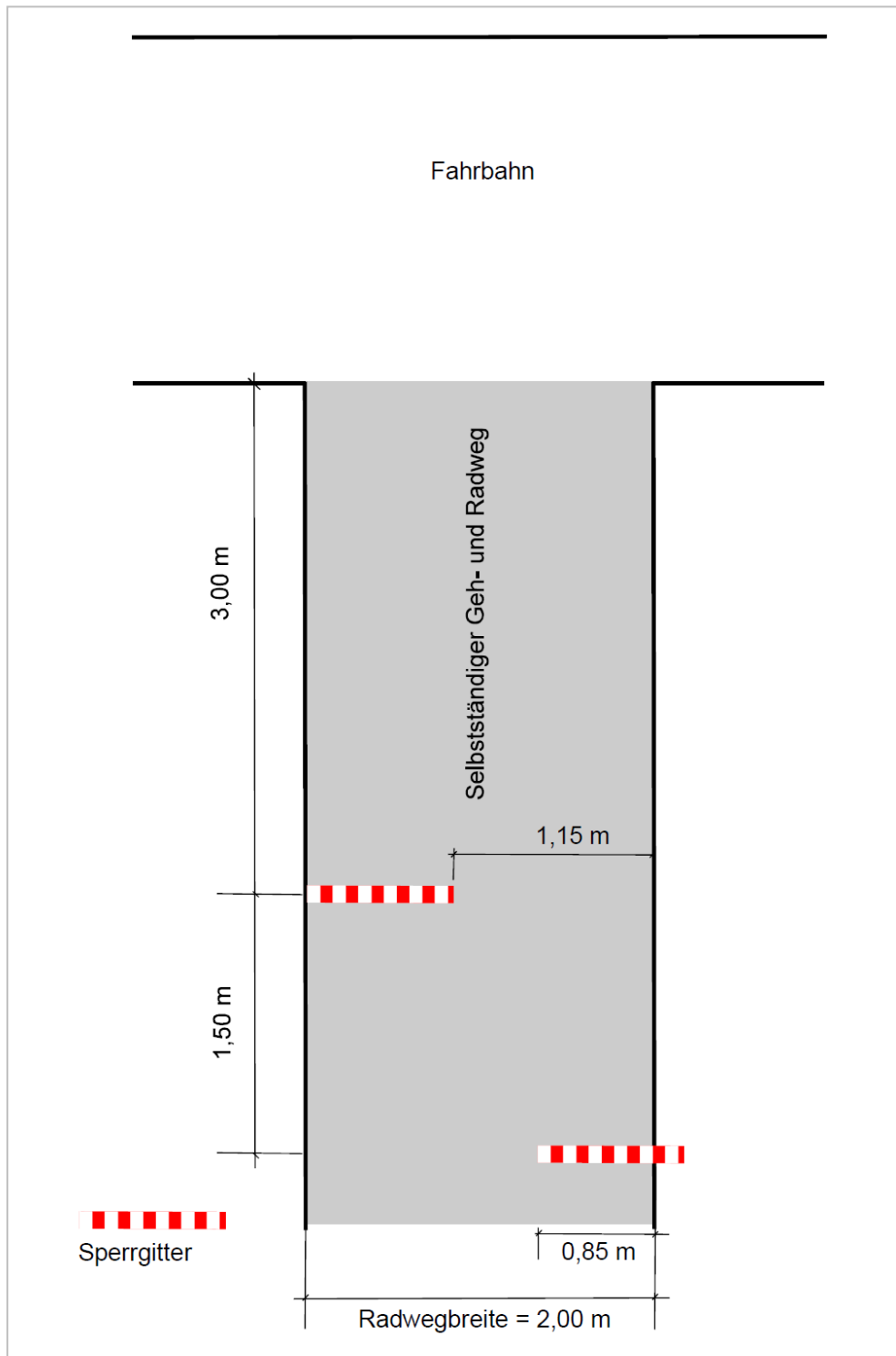
Abb. 16: Installation von Umlaufsperrn gemäß ERA
